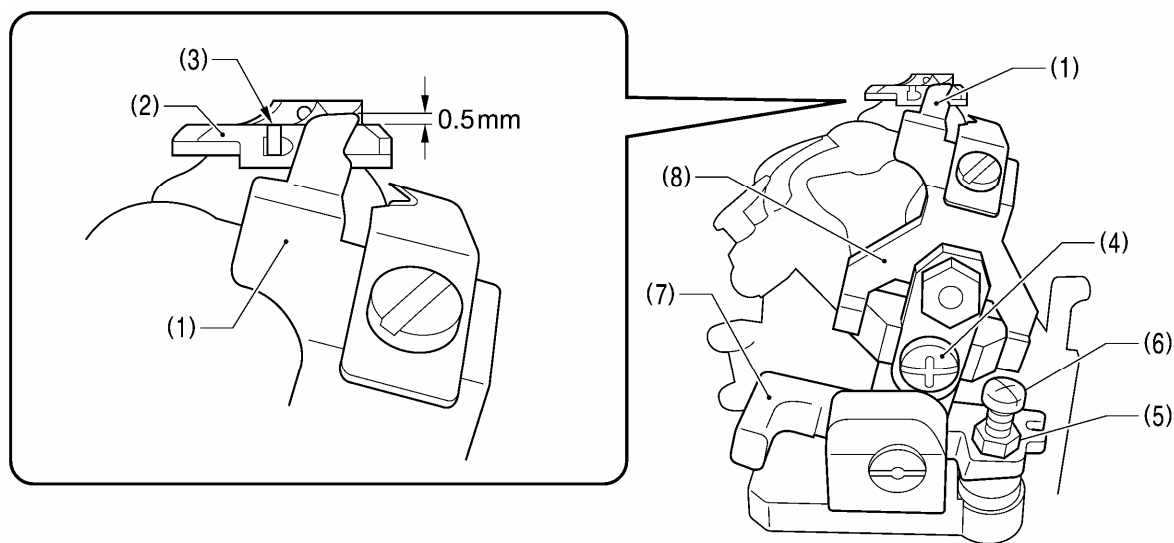
(Вид спереди )
